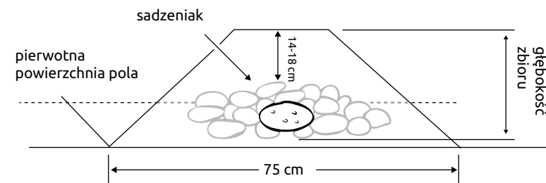
Schemat: Optymalne ułożenie bulw i formowanie rzędów. Pierwotna powierzchnia pola, sadzeniak, głębokość zbioru.
